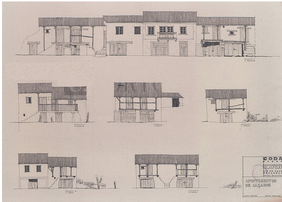
Figura 3.1.14. Sérgio Fernandez, Levantamento, Alçados das casas de Rio de Onor, Recuperação de aldeias em Rio de Onor, 1964, CODA.
