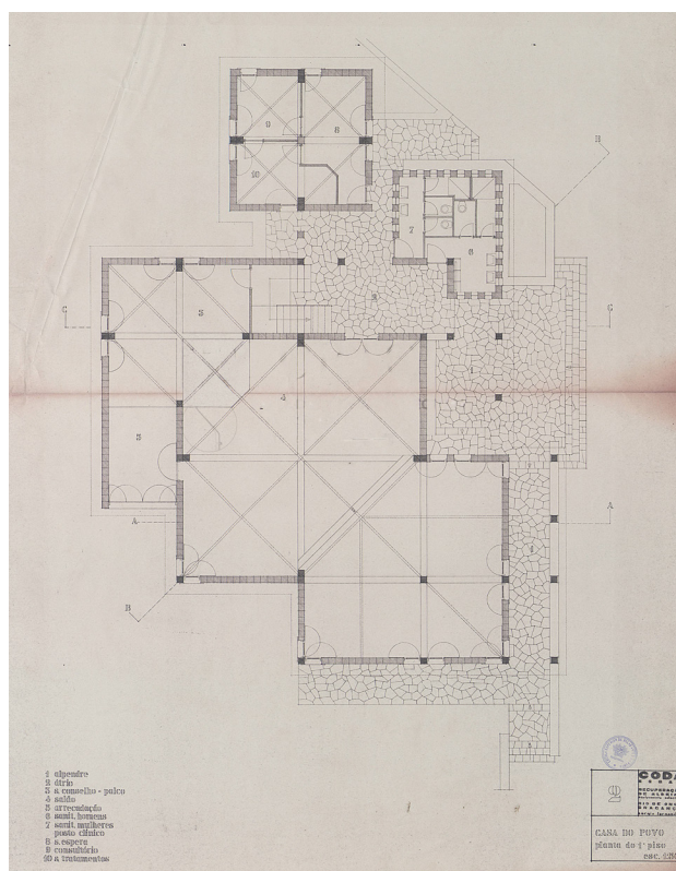
Figura 3.1.18. Sérgio Fernandez, Planta do Projeto para a casa do povo de Rio de Onor , Recuperação de aldeias em Rio de Onor, 1964, CODA.
