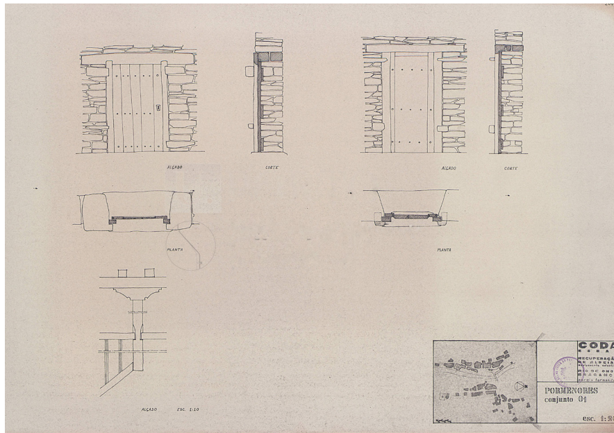
Figura 3.1.11. Sérgio Fernandez, Levantamento, Desenho técnico de detalhes construtivos das construções de Rio de Onor, Recuperação de aldeias em Rio de Onor, 1964, CODA.
