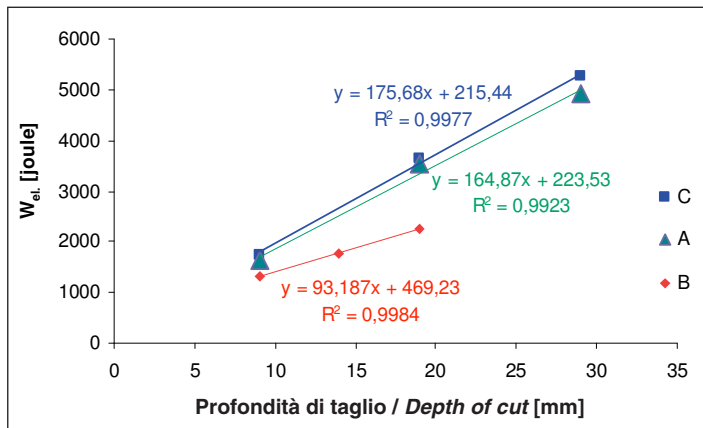
Fig. 7. Relazione tra il consumo di energia elettrica ( W_{el} ) e la profondità del taglio per ognuno degli utensili (A,B,C). Relation between electrical energy consumption ( W_{el} ) and the depth of cut for each of the tools (A, B, C).
